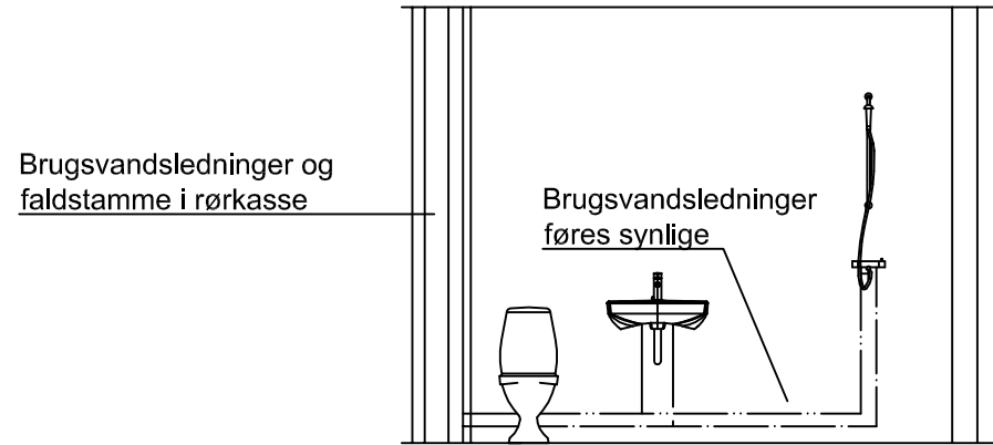
Opstalt, bad
