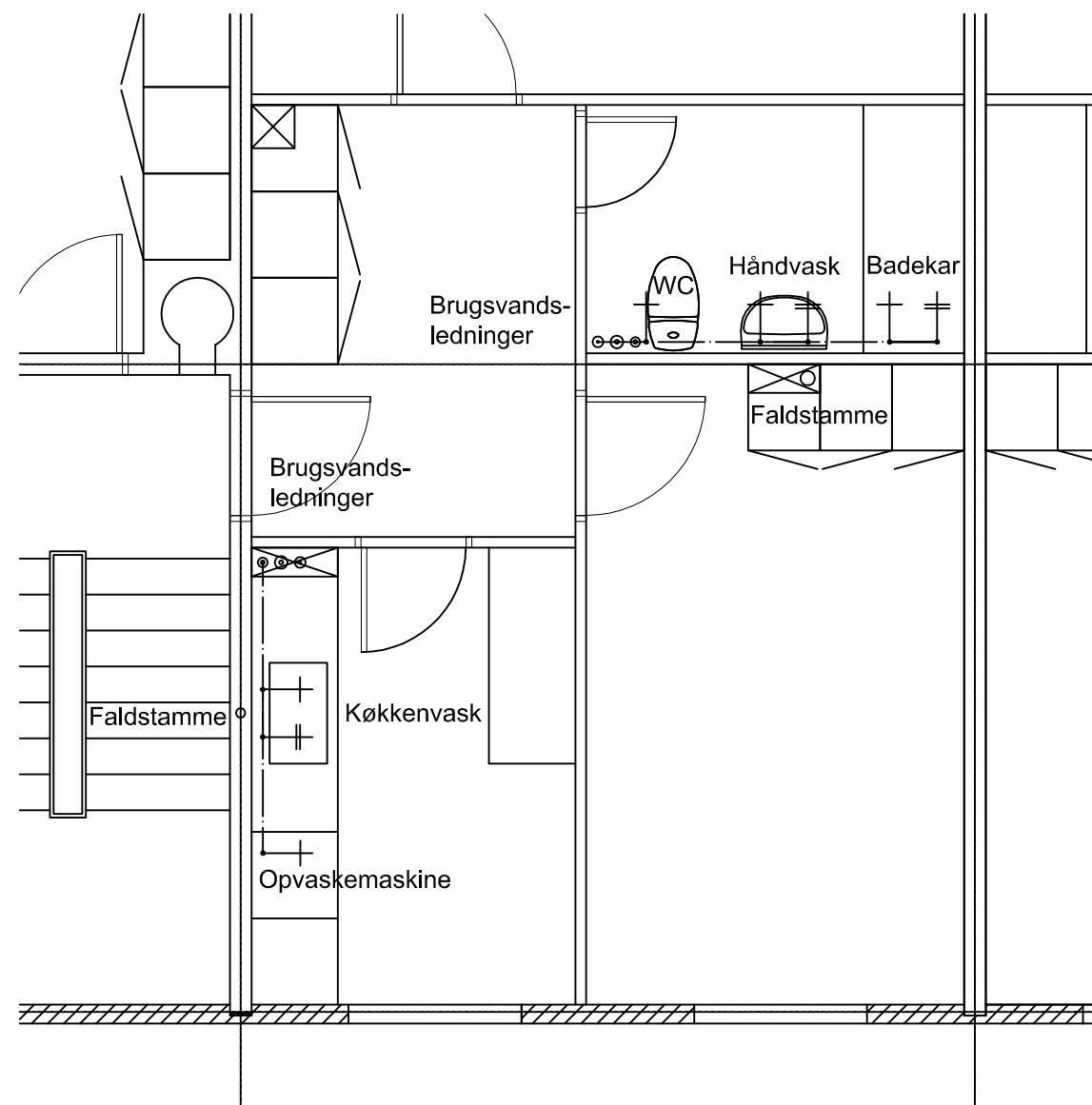
Plan, bad og køkken
